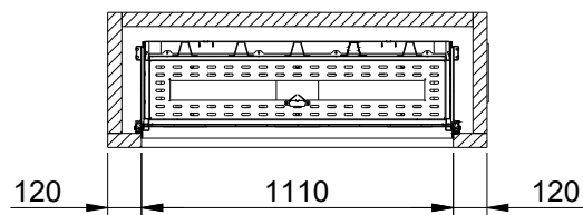
A-A (1:30)
