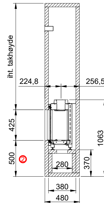
D-D (1:30)
