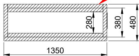
B-B (1:30)
